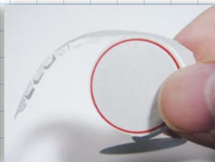
22、タイヤと同じ要領で接着させていきます。
